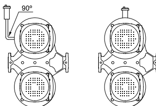
Рис. 7 Автоматический воздухоотводчик
