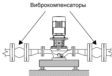
Рис. 11 Насос TP с виброкомпенсаторами большего размера
