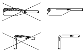
Рис. 9 Правильная конфигурация трубопроводов на стороне всасывания
